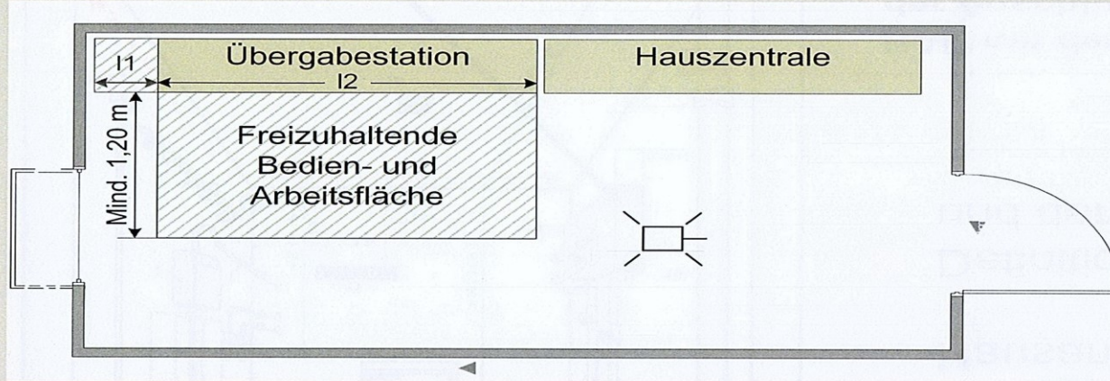
Platzbedarf von Fernwärme-Übergabestationen
